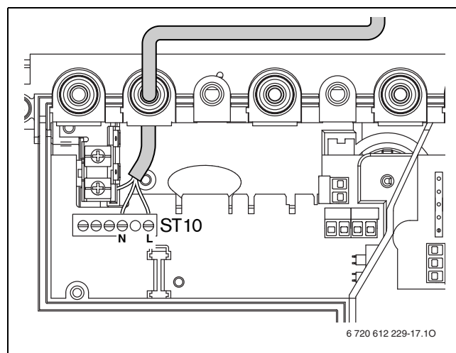
Fig. 29 Morsettiera ST10 per alimentazione di tensione
