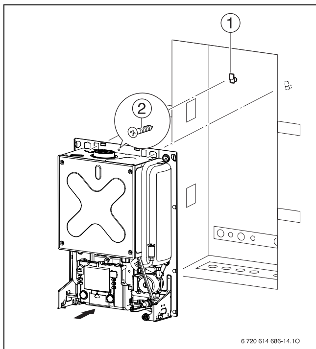
Fig. 12 Fissaggio a parete nel guscio ad incasso
