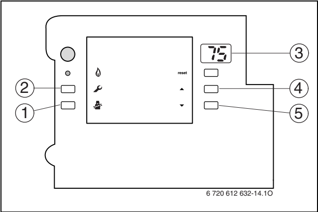
Fig. 37 Panoramica degli elementi operativi
