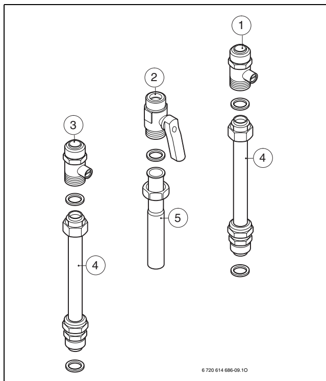
Fig. 16 Set di collegamento
