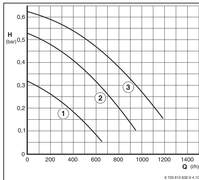
Fig. 36 Diagramma delle curve caratteristiche/velocità del circolatore
