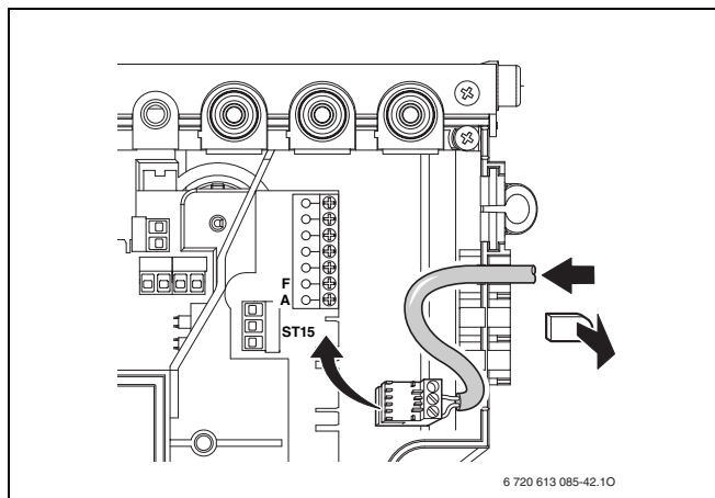
Fig. 27 Collegamento sonda della temperatura del bollitore (NTC)
