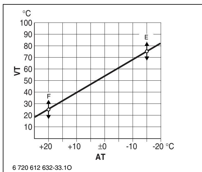
Fig. 34 Curva di riscaldamento
