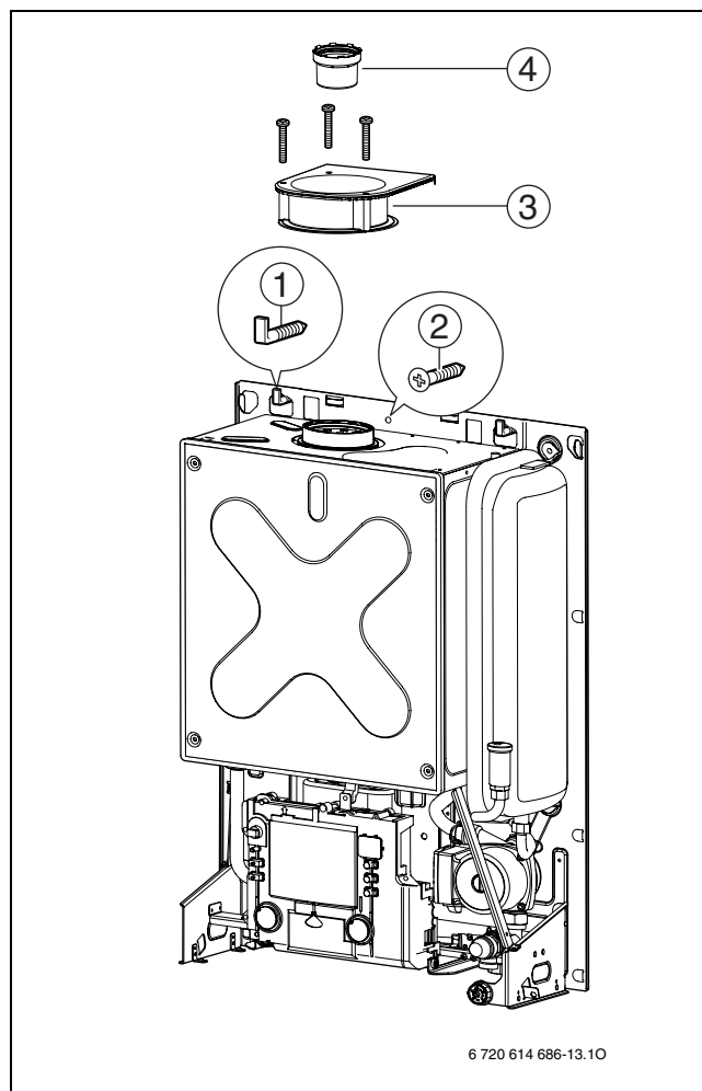
Fig. 11 Fissaggio a parete
