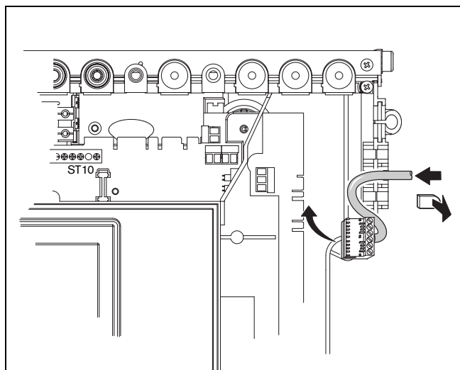
Fig. 26 Collegamento della valvola a tre vie
