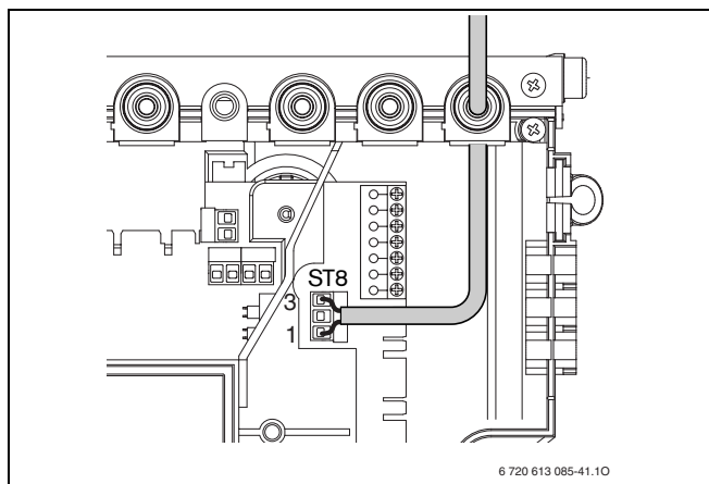
Fig. 28 Collegamento termostato del bollitore
